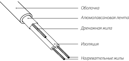
Конструкция кабеля нагревательного WSS
