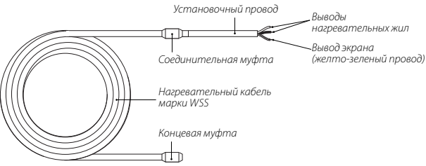
Конструкция кабеля нагревательного WSS
