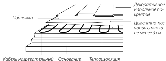
Схема укладки под ламинат, линолеум или ковровин в холодных помещениях
