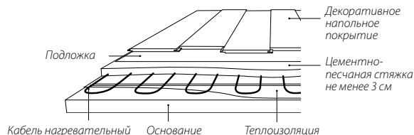
Схема укладки под ламинат, линолеум или ковровин
