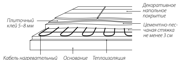
Схема укладки под керамическую плитку в холодных помещениях
